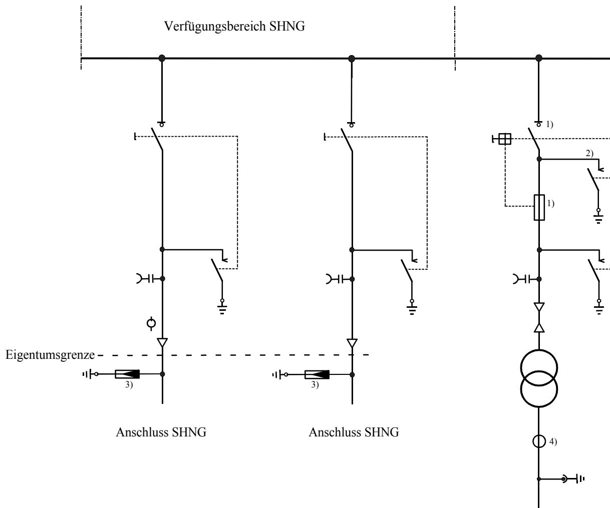
Bild 2. Übergabestation mit einem Transformator, zwei SHNG Anschlussleitungen und niederspannungsseitiger Verrechnungsmessung
