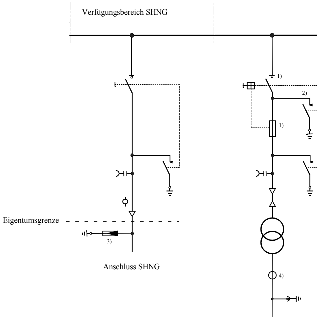
Bild 1. Übergabestation mit einem Transformator, einer SHNG Anschlussleitung und niederspannungsseitiger Verrechnungsmessung
